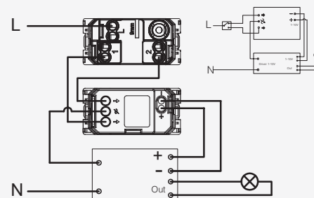
Dimmer 1-10V - Interruptor 2 vías N0160.9 XX
