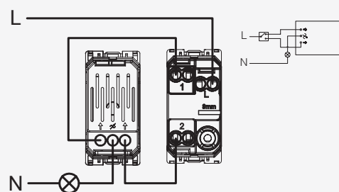
Dimmer - Interruptor 2 vías
